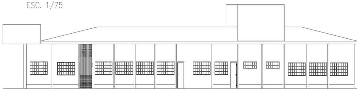
ELEVAÇÃO LATERAL ESC. 1/75
