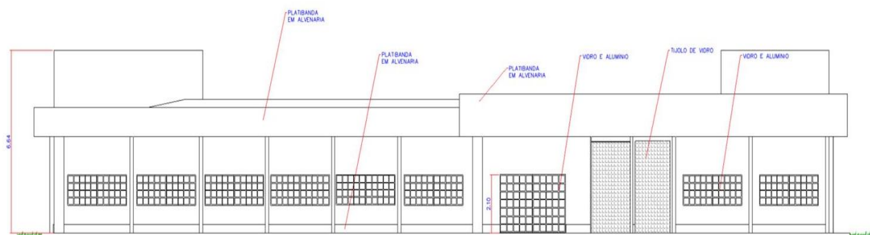
ELEVAÇÃO FRONTAL ESC. 1/75
